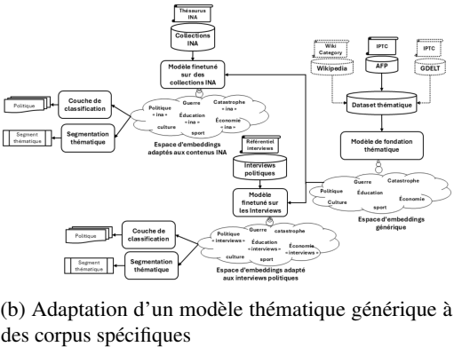
FIGURE 1 – Architecture étendue des modèles proposés
