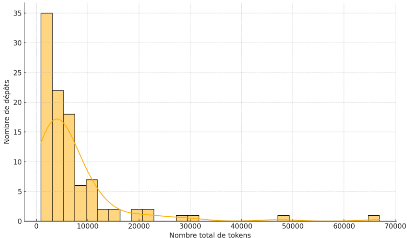
FIGURE 1 – Distribution du nombre total de tokens par dépôt dans RepoTransBench.
