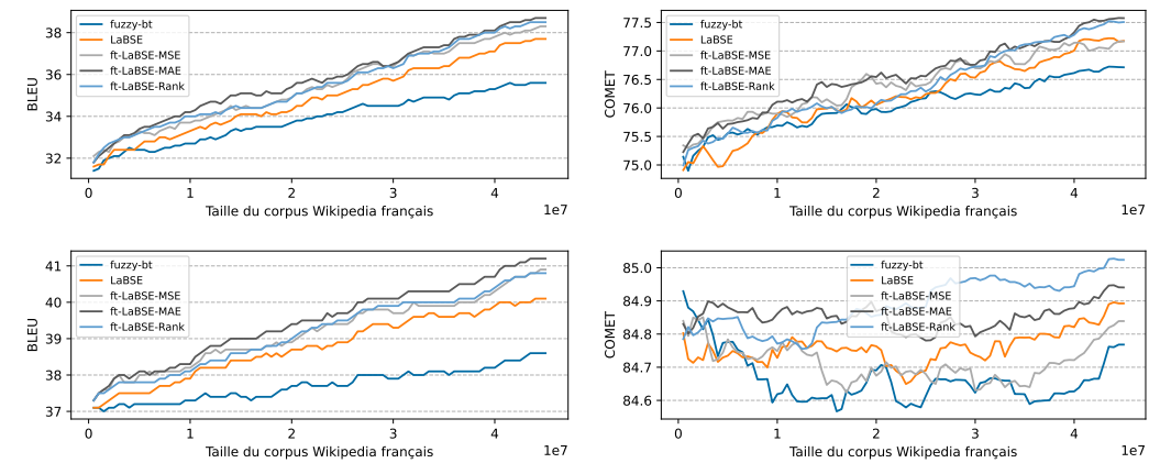
FIGURE 1 – Évolution des scores BLEU et COMET de TM^3 -LevT (en haut) et NFA (en bas) en augmentant la taille du corpus de recherche.
