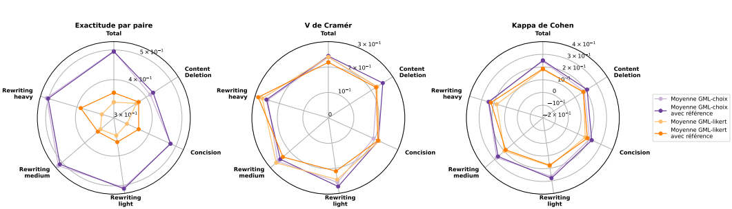
FIGURE 14 – Alignement des approches GML-juge avec les annotations humaines par catégories de révision.
