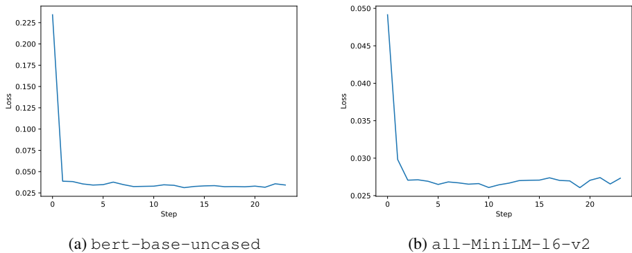
FIGURE 5 – Évolution de la perte de validation des modèles lors de l’affinage sur STSbenchmark
