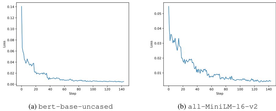
FIGURE 4 – Évolution de la perte d’entraînement des modèles lors de l’affinage sur STSbenchmark
