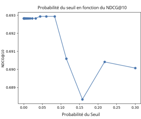
FIGURE 4 – Performance (NDCG@10) sur Sci-Fact en fonction du seuil \theta sur la matrice de coexistence.
