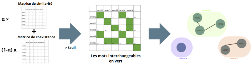
FIGURE 1 – Illustration du processus de clustering des mots
