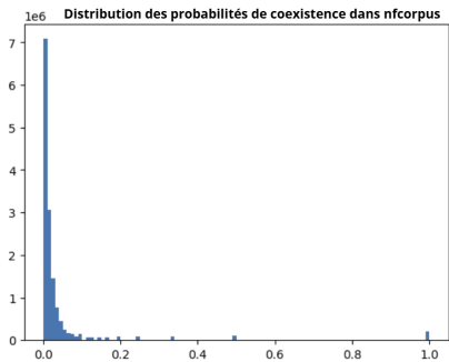
FIGURE 5 – Distribution des probabilités de coexistence dans NFCorpus.
